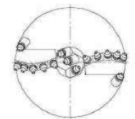
BSZS lišty s výměnnými zuby+pilot s VZ
